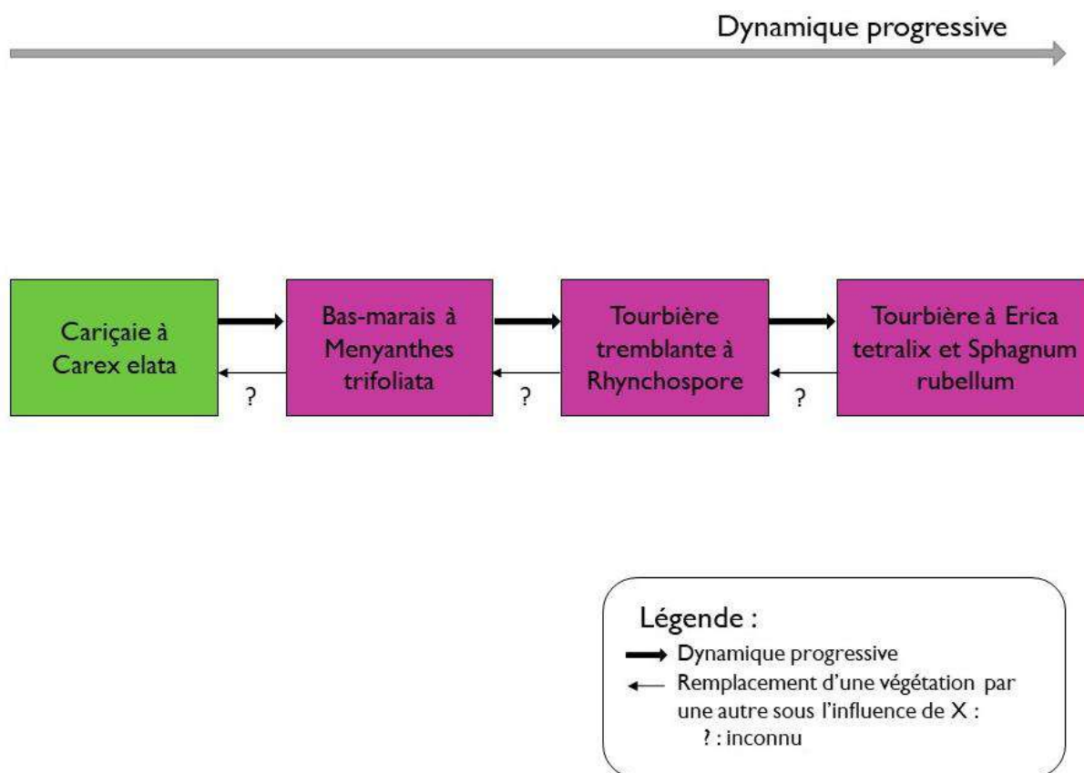
Figure 49 : Schéma du complexe tourbeux oligotrophe humide
