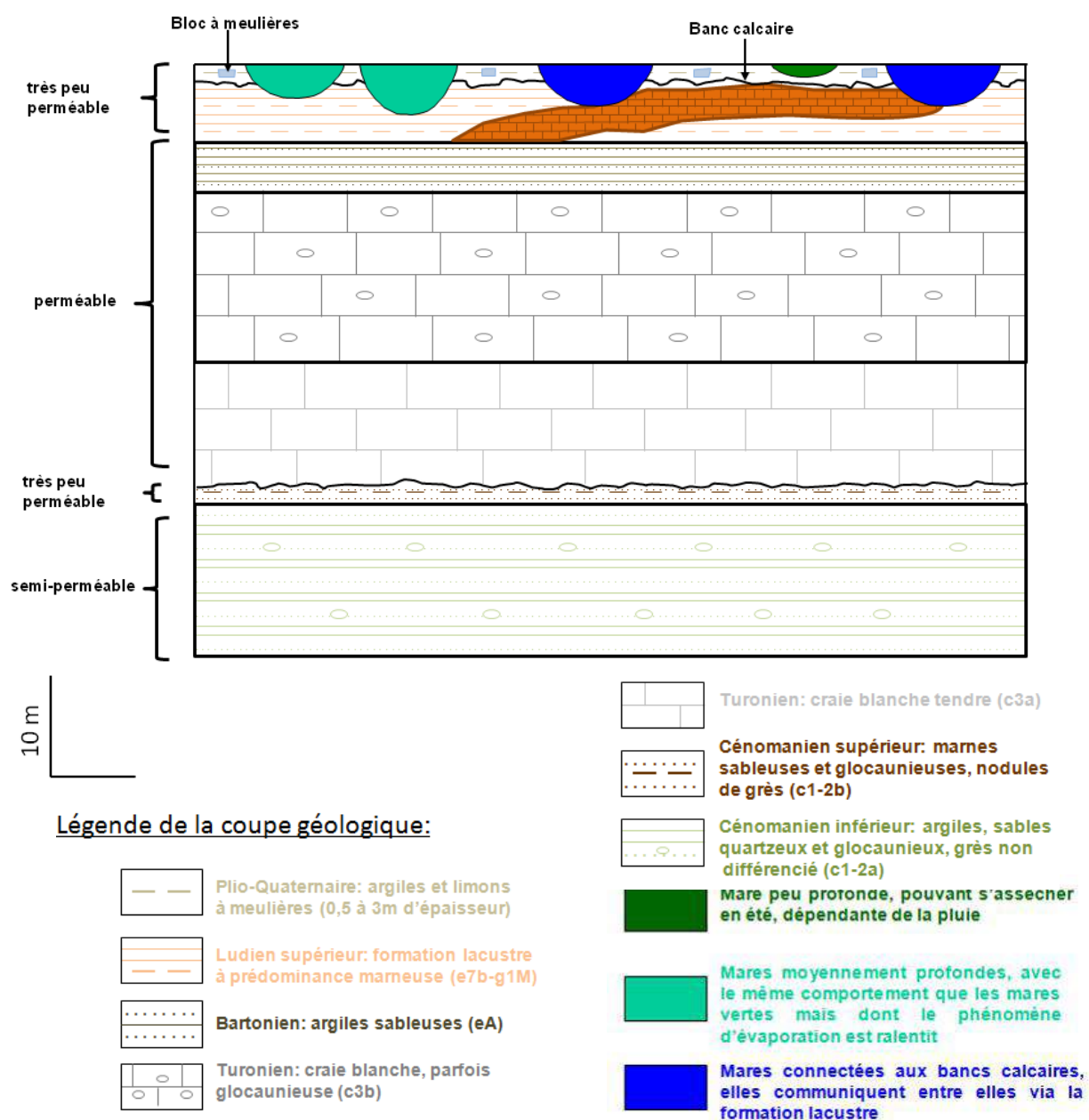
Figure 7 : Coupe stratigraphique du sol de la Réserve du Pinail (source Romain Guibeneuf)
