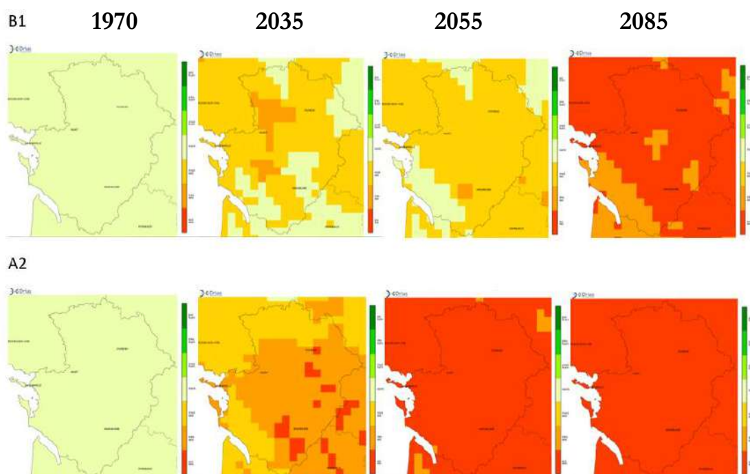
Figure 5 : Simulation de l'indicateur sécheresse d'humidité du sol (SSWT) du modèle ISBA (moyenne annuelle) à partir de la période de référence (autour de 1970).
