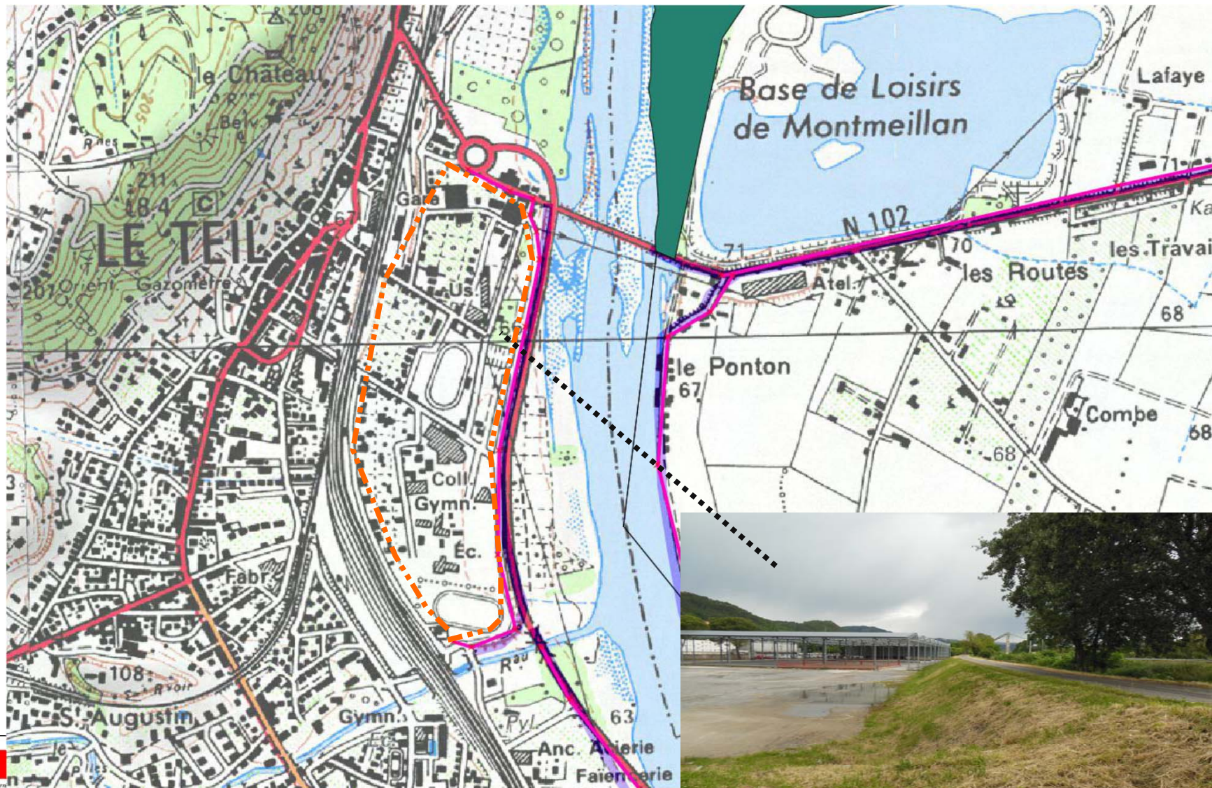
Digue du Frayol (Le Teil – 07) Fermeture amont du système par la RN102
