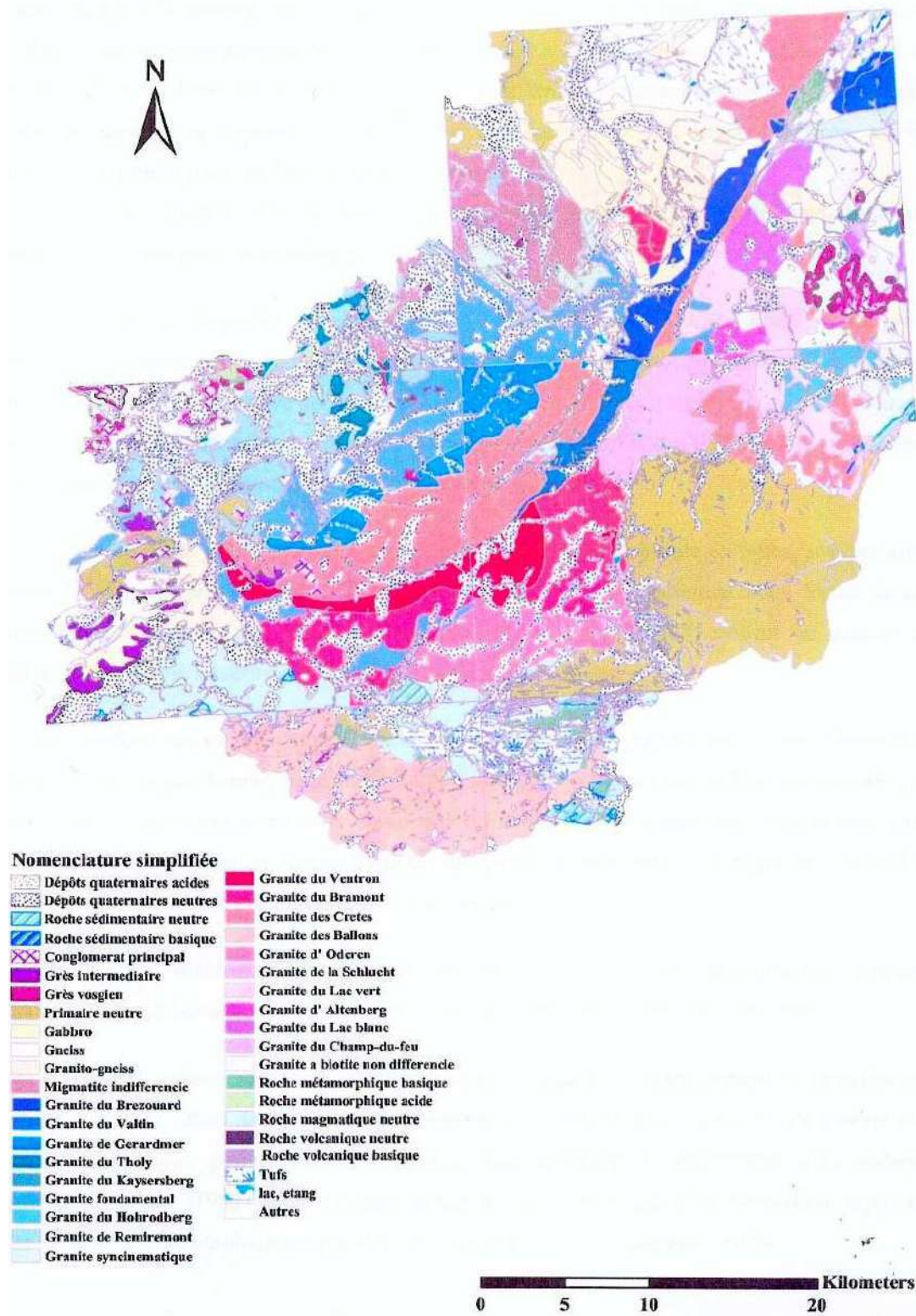
Figure II.2.a : Géologie des Vosges du sud (d'après Nedeltcheva 2005)
