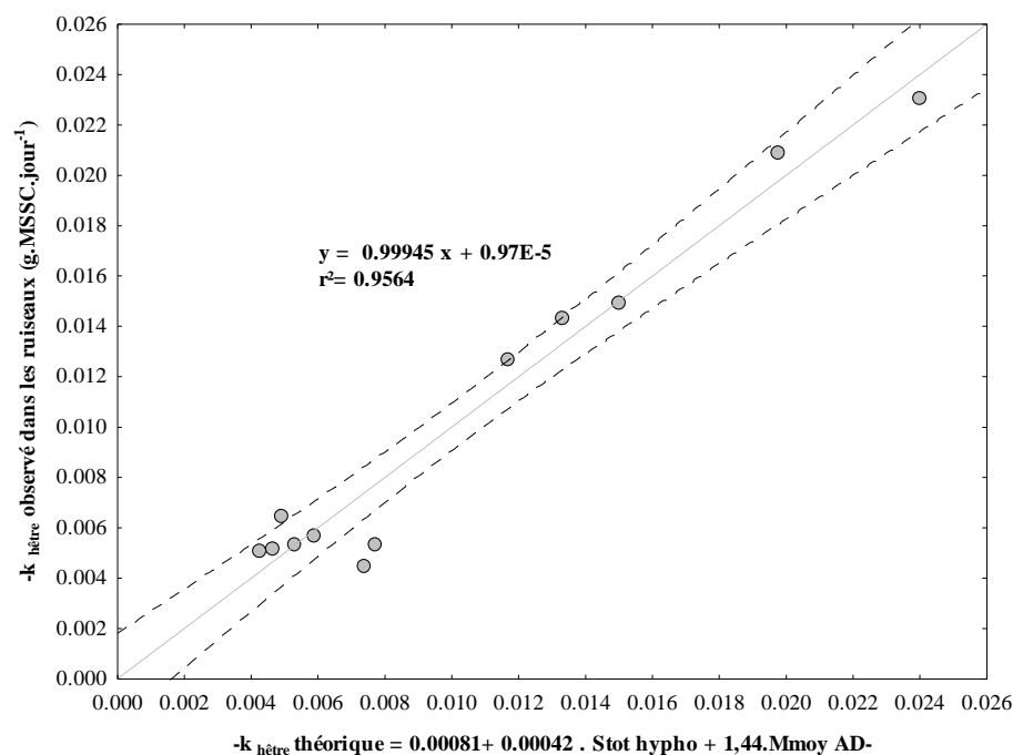
Figure VI.3 : Régression entre le taux de décomposition linéaire des feuilles de hêtre mesuré dans les ruisseaux ( -k observé) et le taux de décomposition théorique ( -k théorique) proposé par le modèle de régression pas à pas, basé sur la diversité des hyphomycètes et la biomasse moyenne des décheteteurs AD- associés aux litières. Les lignes pointillées représentent l'intervalle de confiance à 95%.
